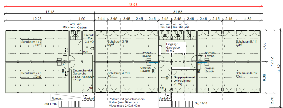
Abb. 3 Regelgeschoss Provisorium 1
