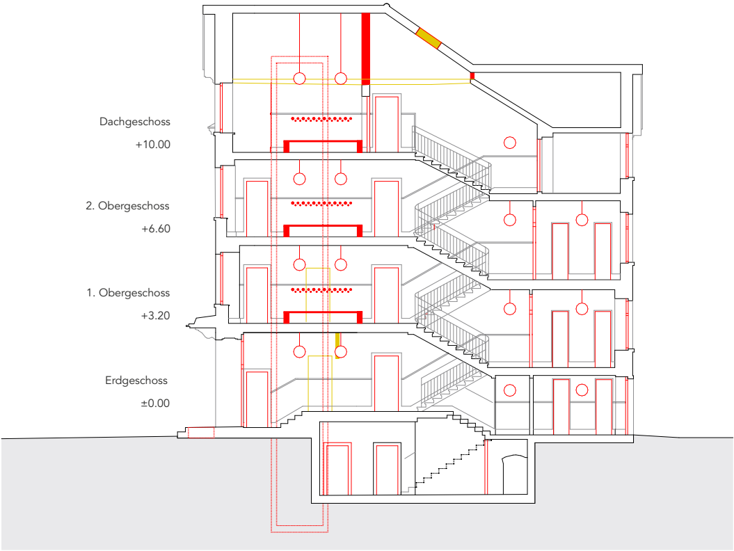
Querschnitt Umbau
