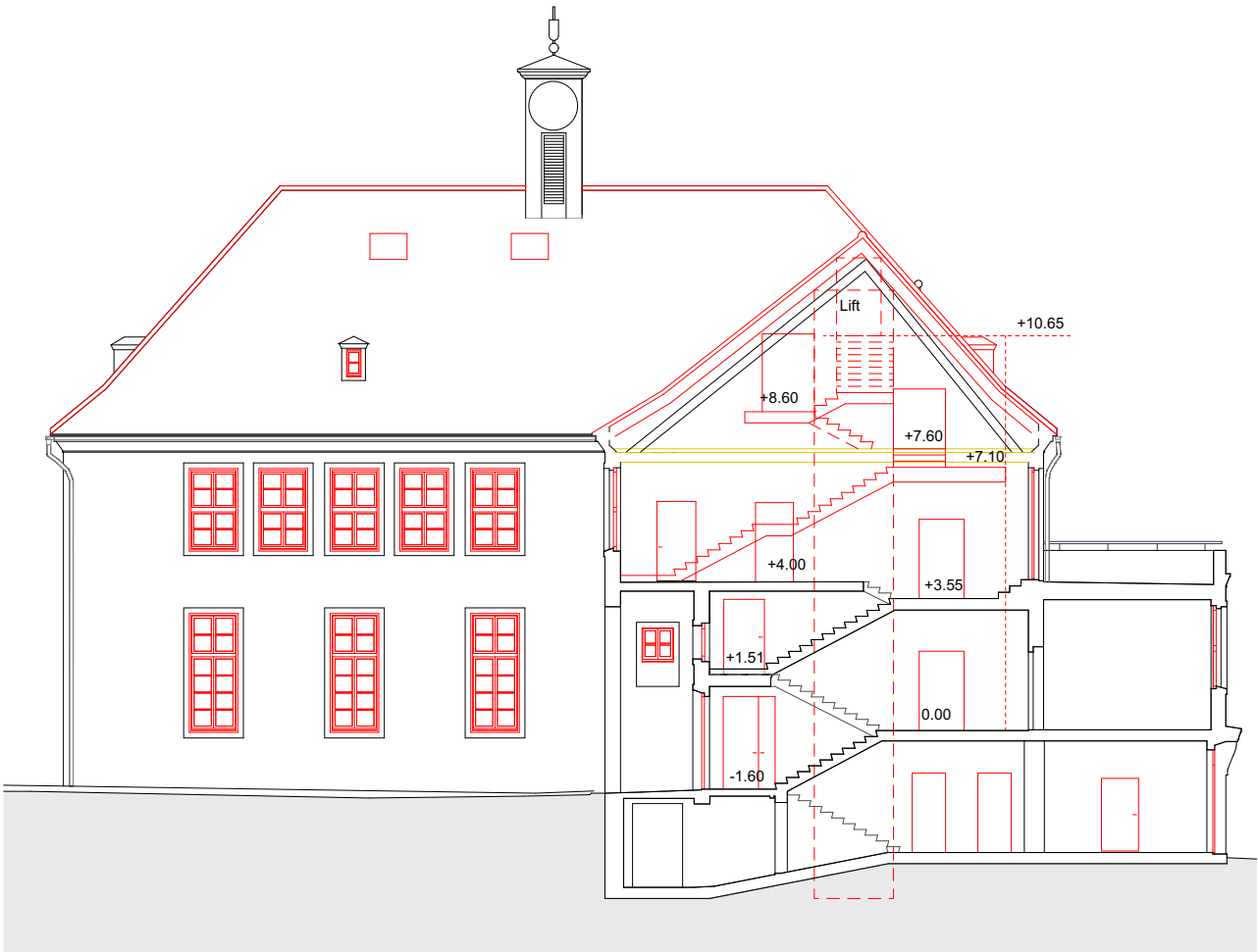
Querschnitt Umbau Zwischenbau
