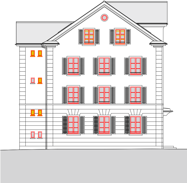
Ansicht Nordwest
