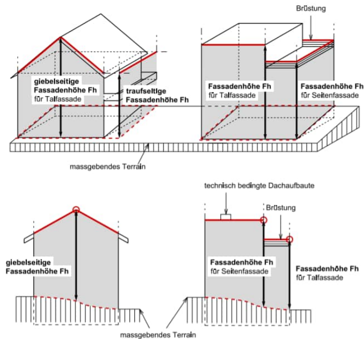
Abbildung 60: Skizze zur Fassadenhöhe (§ 278 PBG), Anhang zur Allgemeinen Bauverordnung (erläuternde Skizzen für die Mess- und Berechnungsweisen gemäss PBG und ABV ZH)
