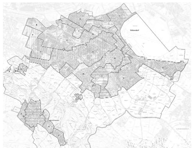
Abbildung 245: ÖV-Güteklasse-Plan der revidierten Verordnung über die Fahrzeugabstellplätze
