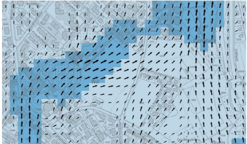
Abbildung 86: Kaltluftvolumenstrom im Bereich der Gestaltungspläne Schönggrundstrasse und Chrummacherstrasse, Klimaanalysekarte GIS ZH
